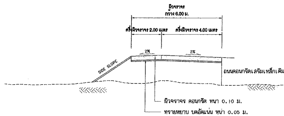
รูปตัดแสดงโครงสร้างถนนคอนกรีต
