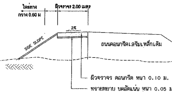
รูปตัดแสดงโครงสร้างถนนคอนกรีต
